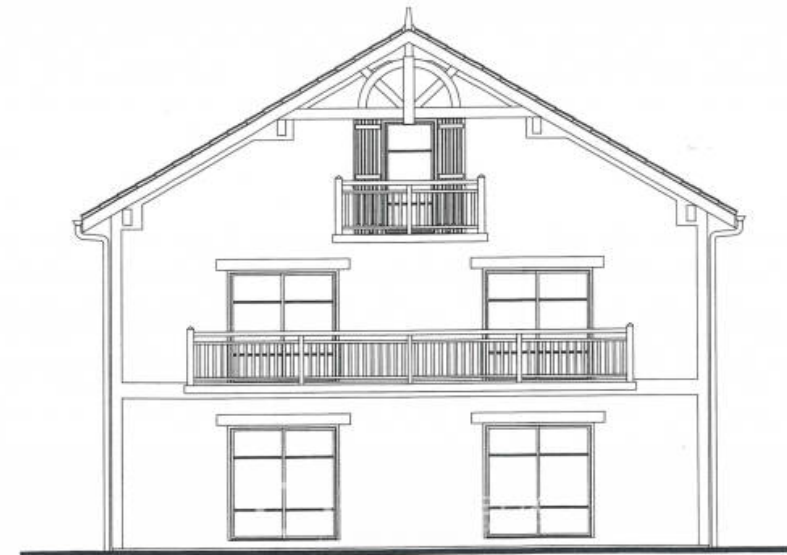
FACADE SUD-OUEST
