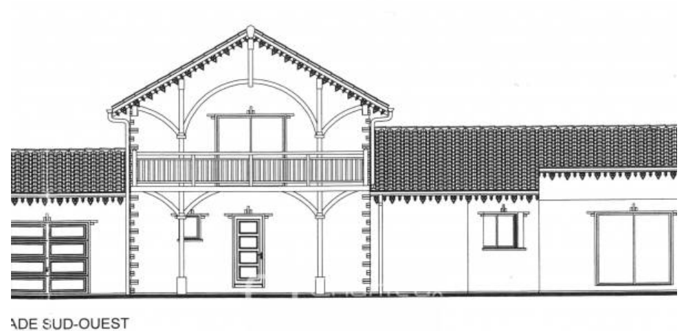
FAÇADE SUD-OUEST
